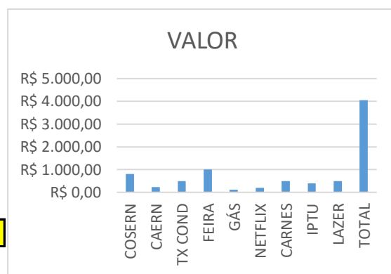
FUNÇÕES ESTATÍSTICAS
